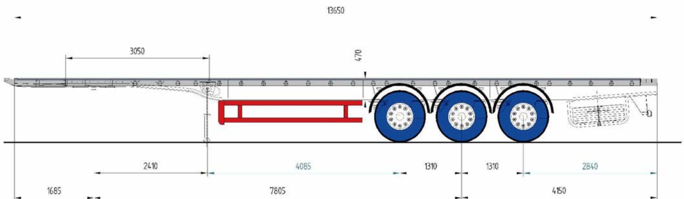
Plataforma aluminio. Modelo: PTR-136-3 Ejes.
