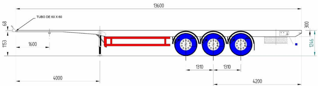
Chasis de frigorífico. Modelo: ENF - 3 Ejes.
