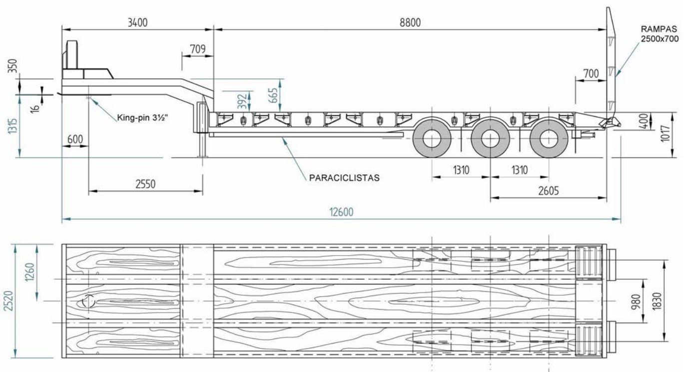
Góndola acero. Modelo: CT57—3 ejes.
