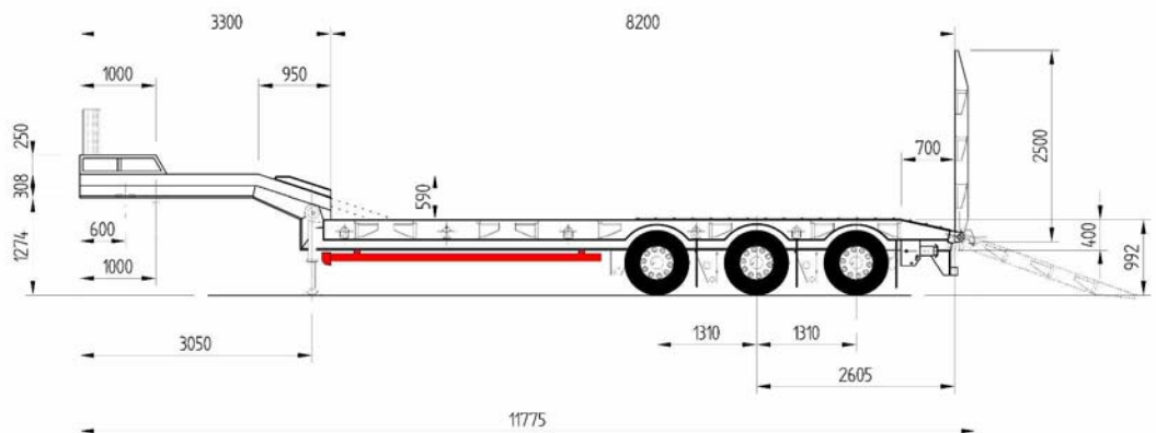
Gondola. Modelo: CT-3 Ejes.
