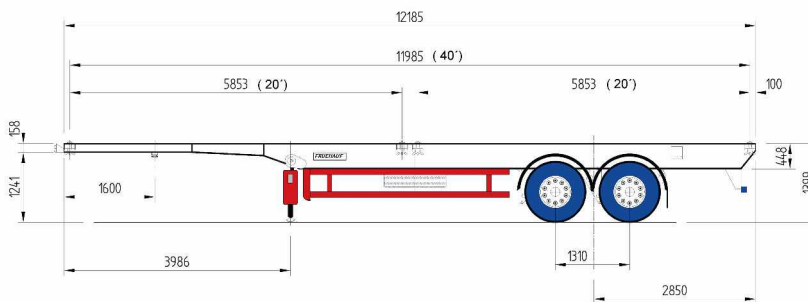
Chasis portacontenedor. Modelo: KNB-122-2 Ejes.
