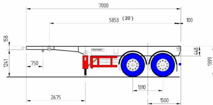
Chasis portacontenedor. Modelo: KNB-70-2 Ejes.
