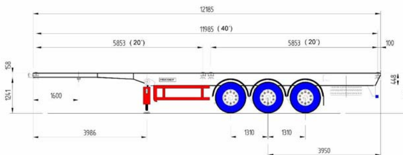
Chasis portacontenedor. Modelo: KNB-122-3 Ejes.
