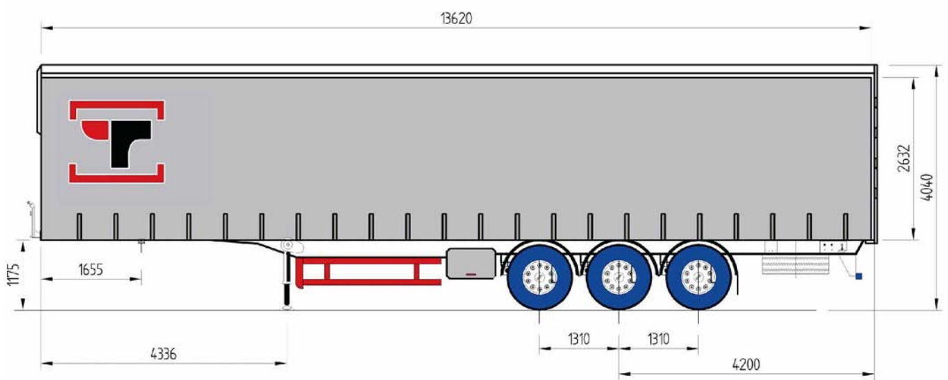
Plataforma acero. Modelo: LMT-136—3 ejes.
