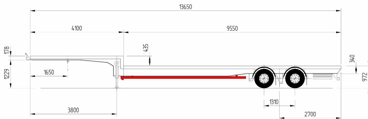
PBD-B6 - 2 ejes.
