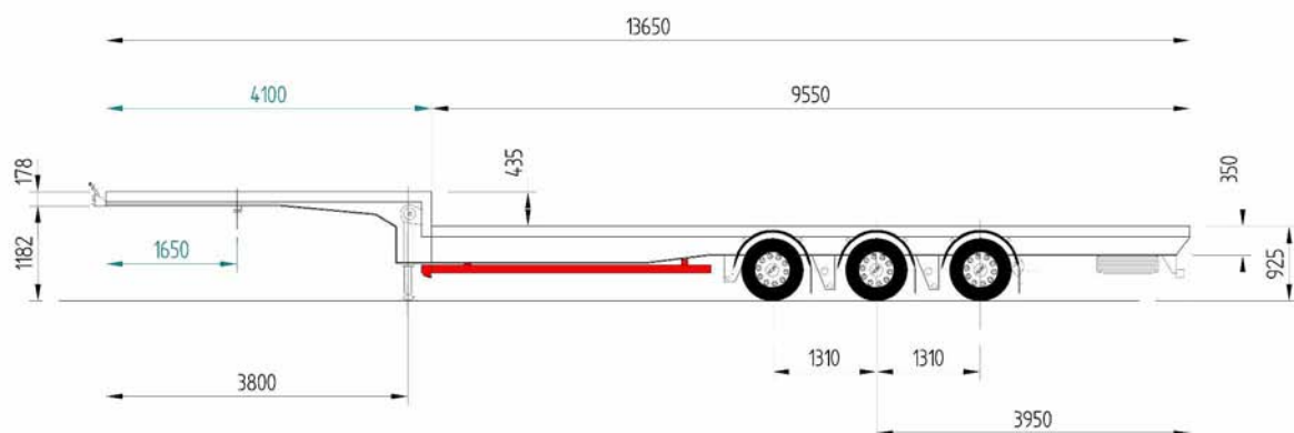
PBD-B6 - 3 ejes.
