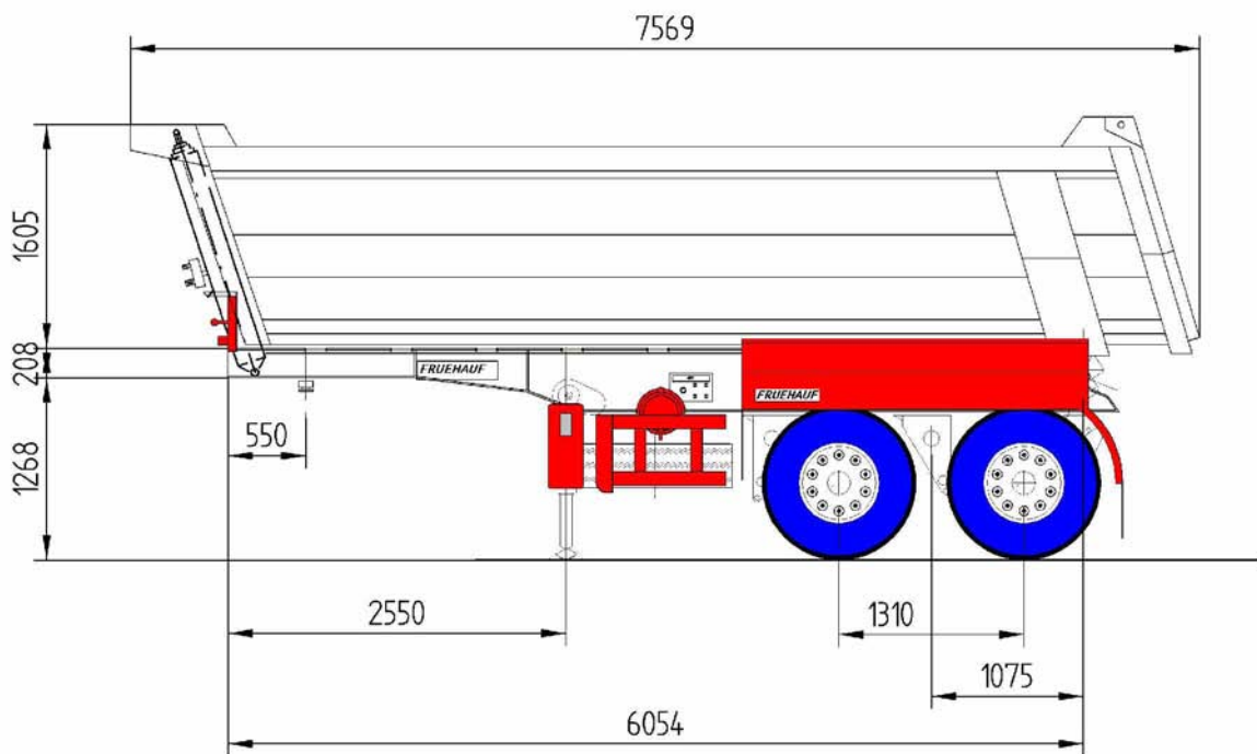
YCHP-73/20 - 2 ejes.
