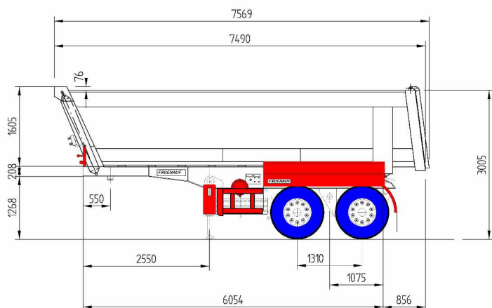
YCH-73/20 - 2 ejes.
