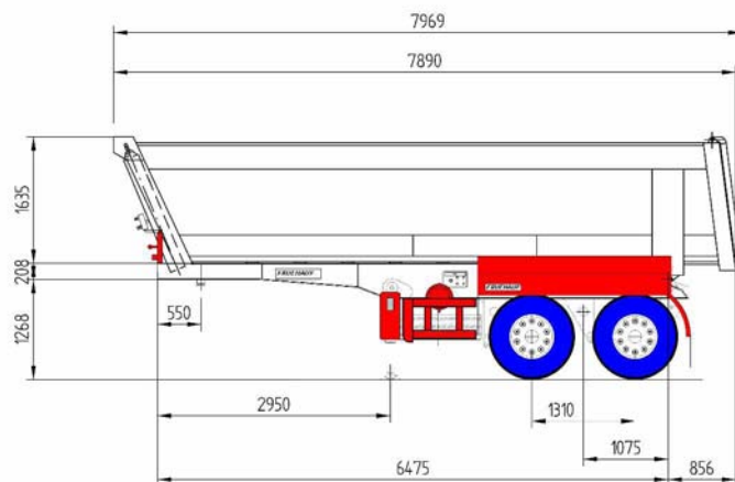
YCH-76/20 - 2 ejes.
