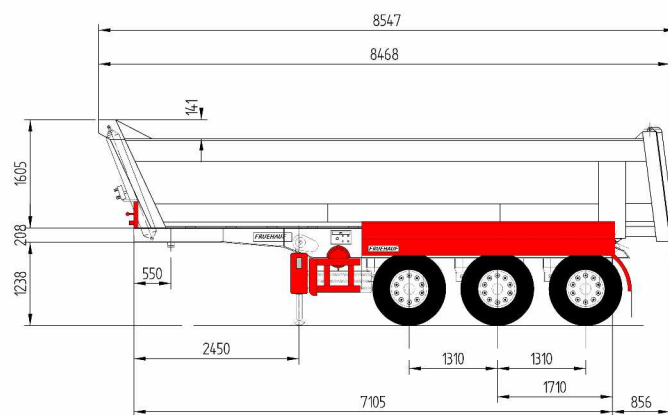
YCH-85/25 - 3 ejes.
