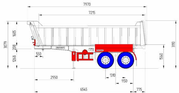
YBH-76/20-2 ejes. Frente Plano.
