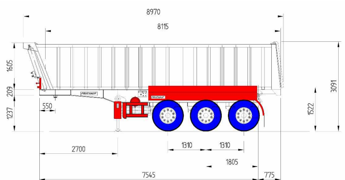
YBH-85/25-3 ejes. Frente Plano.
