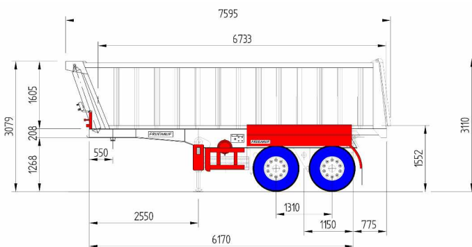
YBH-73/20-2 ejes. Frente Plano
